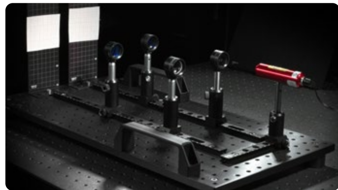
Kit pédagogique de collimation laser
